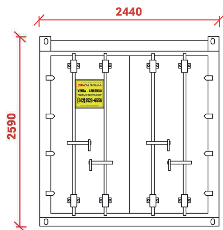
Elevación Este
