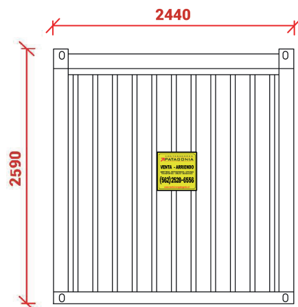
Elevación Oeste
