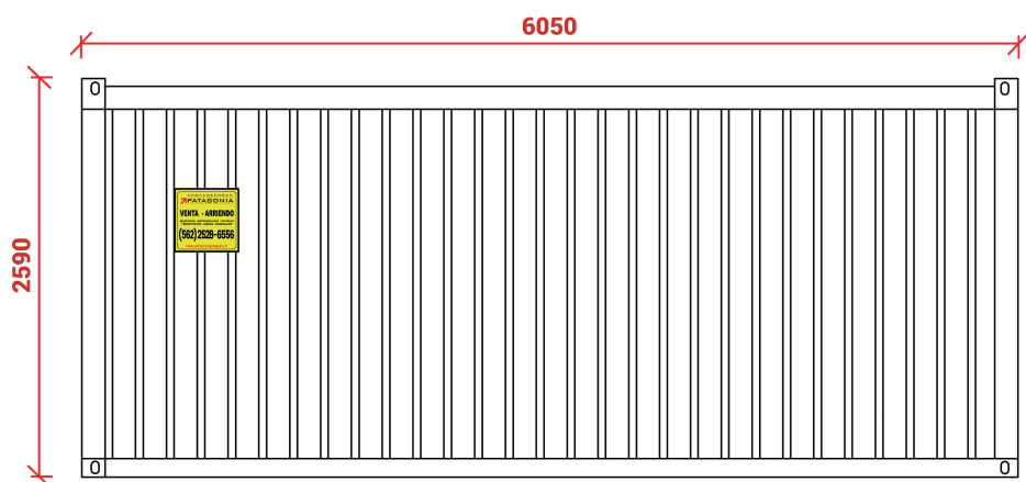
Elevación Sur
